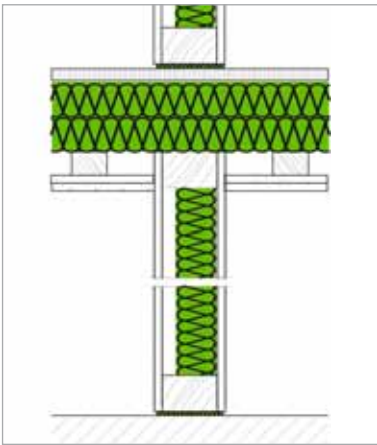
ANSCHLUSS AN HOLZBALKENDECKE
