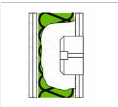
EINBAU STECKDOSE MIT GIPSMÖRTEL
